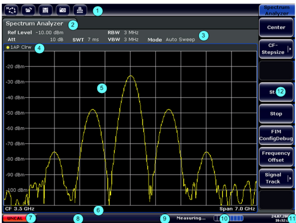
图 5-1: 分析仪操作过程中 R&S FSV 的屏幕布局
