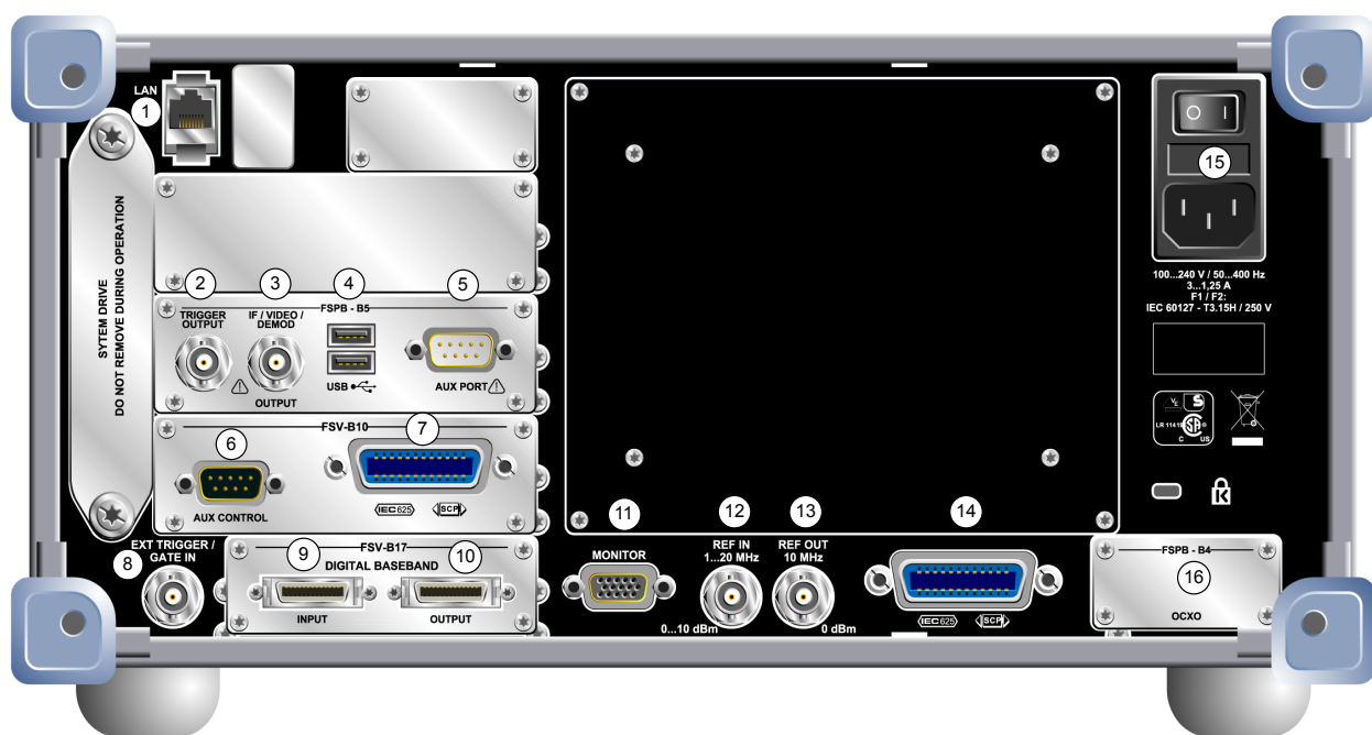
图 2-3: 后面板视图
