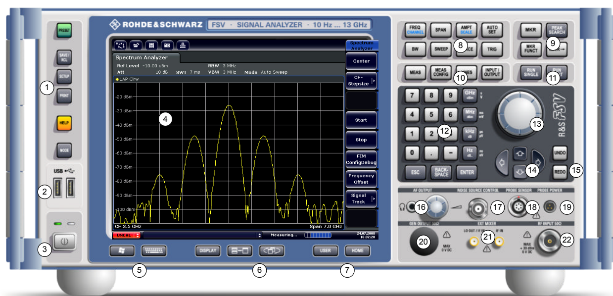
图 2-1: 前面板视图
